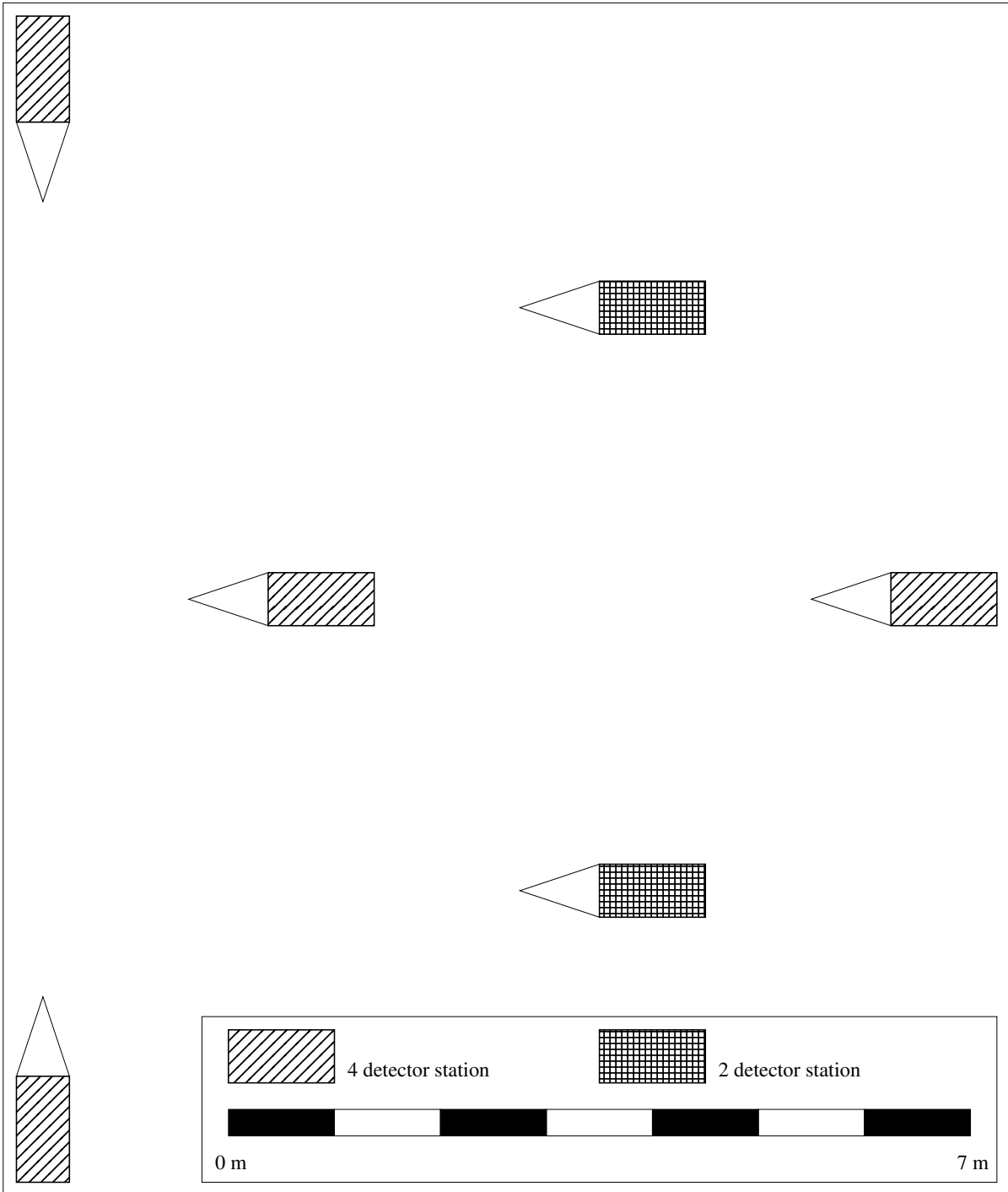
Figuur 2.2 – Meetstations
